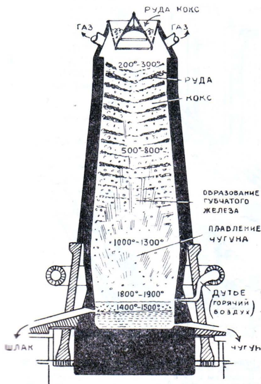
Разрез доменной печи.
