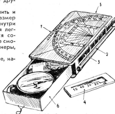
Рисунок 1. (1 — на этой стороне пенала расположен солнечный высотмер; 2 — трубочка; 3 — линейка дальсмера; 4 — крышка с «лесенкой»; 5 — крышка с отверстием; 6 — коробочка с компасом, курвиметром и др.).
